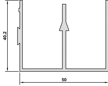
4633 AĞIRLIK / WEIGHT 0,810 kg/m
