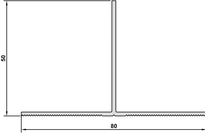
4216 AĞIRLIK / WEIGHT 0,553 kg/m
