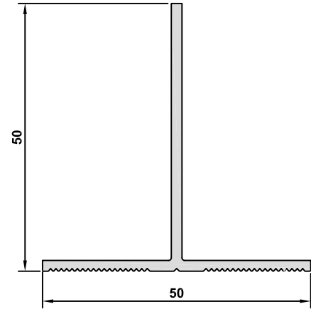
6374 AĞIRLIK / WEIGHT 0,510 kg/m
