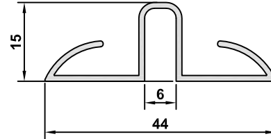
6640 AĞIRLIK / WEIGHT 0,280 kg/m
