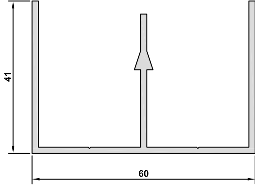
4653 AĞIRLIK / WEIGHT 0,827 kg/m
