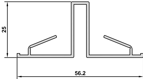
4668 AĞIRLIK / WEIGHT 0,428 kg/m
