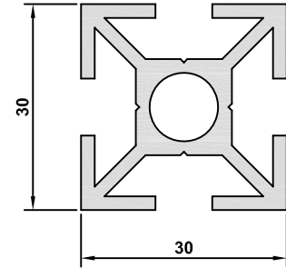
5426-2.0 AĞIRLIK / WEIGHT 0,930 kg/m
