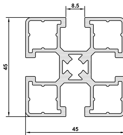
7773 AĞIRLIK / WEIGHT 1,442 kg/m
