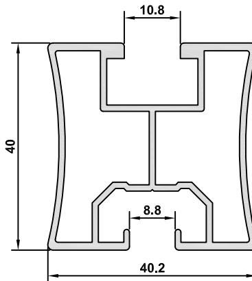
7597 AĞIRLIK / WEIGHT 0,840 kg/m
