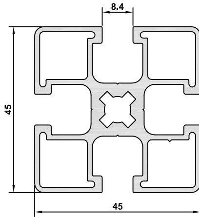
7773 AĞIRLIK / WEIGHT 1,442 kg/m
