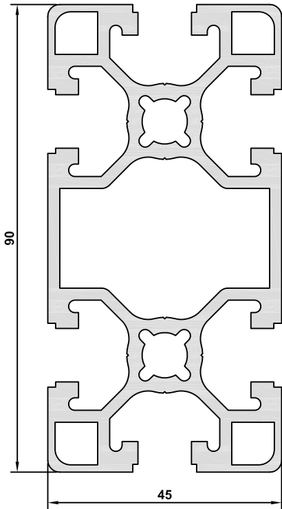
8579 AĞIRLIK / WEIGHT 3,190 kg/m
