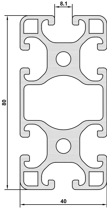
2435 AĞIRLIK / WEIGHT 2,981 kg/m
