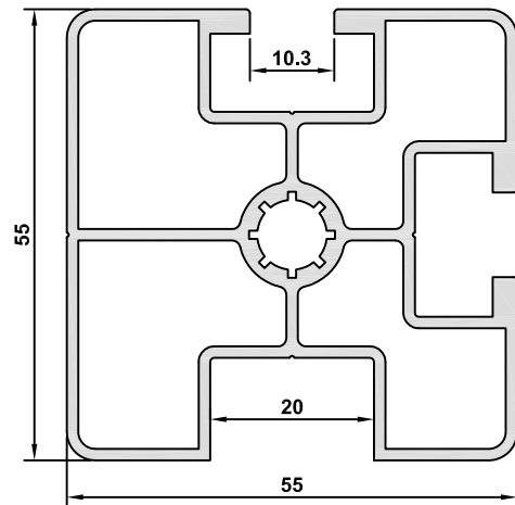
6670 AĞIRLIK / WEIGHT 1,572 kg/m
