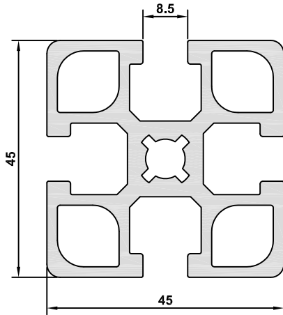
7831 AĞIRLIK / WEIGHT 1,984 kg/m
