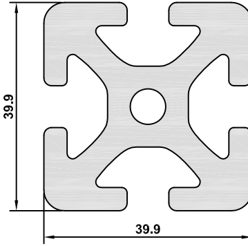
9279 AĞIRLIK / WEIGHT 2,500 kg/m
