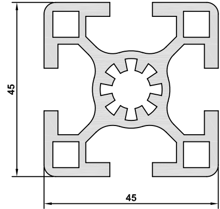
4652-1.8 AĞIRLIK / WEIGHT 2,000 kg/m
