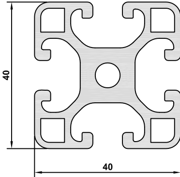
8528 AĞIRLIK / WEIGHT 1,694 kg/m
