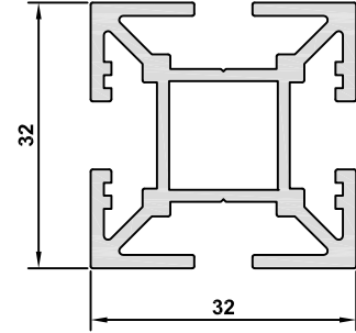
NOV-899 AĞIRLIK / WEIGHT 0,870 kg/m
