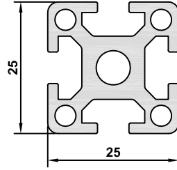
9226 AĞIRLIK / WEIGHT 0,792 kg/m
