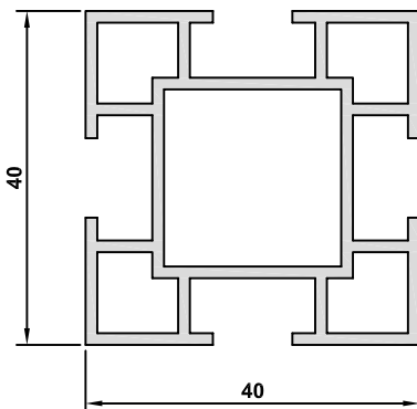
2073-1.4 AĞIRLIK / WEIGHT 0,987 kg/m
