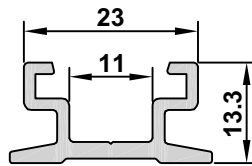
20302 AĞIRLIK / WEIGHT 0,301 kg/m
