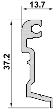
EHS-80 AĞIRLIK / WEIGHT 0,344 kg/m
