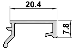
EHS-42 AĞIRLIK / WEIGHT 0,170 kg/m
