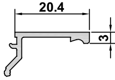
EHS-40 AĞIRLIK / WEIGHT 0,144 kg/m
