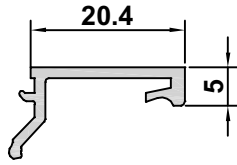
EHS-41 AĞIRLIK / WEIGHT 0,160 kg/m
