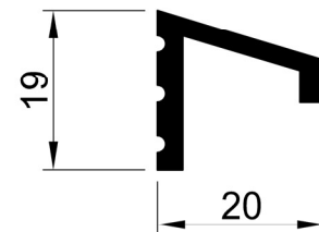
89-108 AĞIRLIK:0.262 kg/mt.
