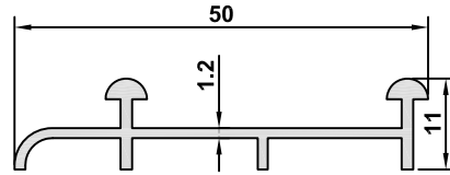
5994 AĞIRLIK / WEIGHT 0,287 kg/m
