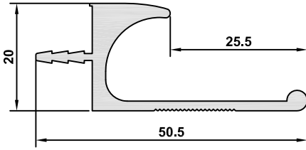
6205 AĞIRLIK / WEIGHT 0,523 kg/m
