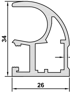
5788 AĞIRLIK / WEIGHT 0,648 kg/m
