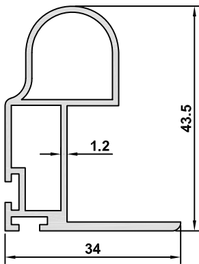
5296 AĞIRLIK / WEIGHT 0,555 kg/m
