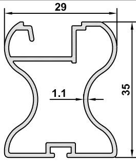
6270 AĞIRLIK / WEIGHT 0,464 kg/m
