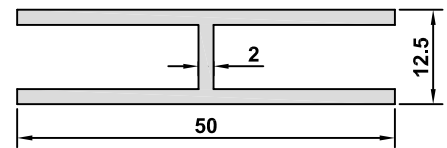
5529 AĞIRLIK / WEIGHT 0,588 kg/m
