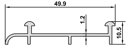
6706 AĞIRLIK / WEIGHT 0,273 kg/m
