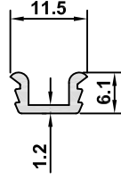
5145 AĞIRLIK / WEIGHT 0,076 kg/m
