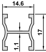
4880 AĞIRLIK / WEIGHT 0,157 kg/m
