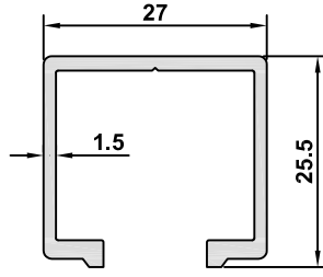
5140 AĞIRLIK / WEIGHT 0,393 kg/m
