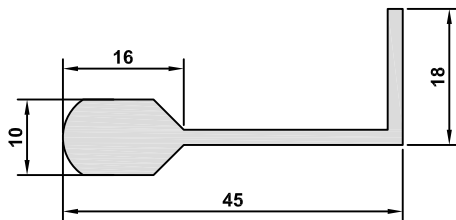
5089 AĞIRLIK / WEIGHT 0,613 kg/m
