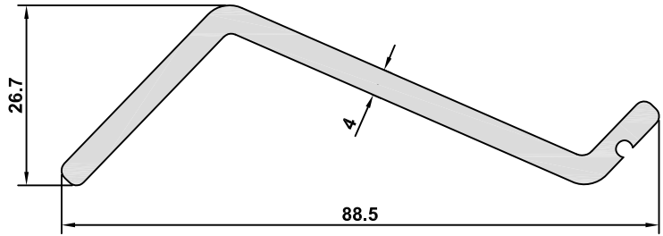
5250 AĞIRLIK / WEIGHT 4,515 kg/m
