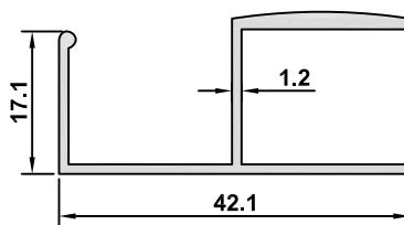
6616 AĞIRLIK / WEIGHT 0,342 kg/m
