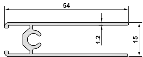
5441 AĞIRLIK / WEIGHT 0,466 kg/m
