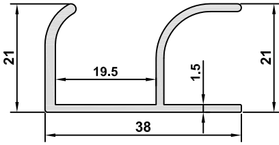
5123 AĞIRLIK / WEIGHT 0,390 kg/m
