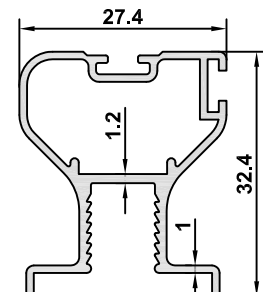
6978 AĞIRLIK / WEIGHT 0,406 kg/m
