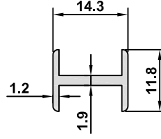
6366 AĞIRLIK / WEIGHT 0,133 kg/m
