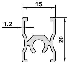
4882 AĞIRLIK / WEIGHT 0,252 kg/m
