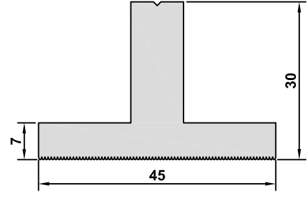
4486 AĞIRLIK / WEIGHT 1,458 kg/m
