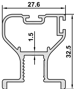
5987 AĞIRLIK / WEIGHT 0,466 kg/m
