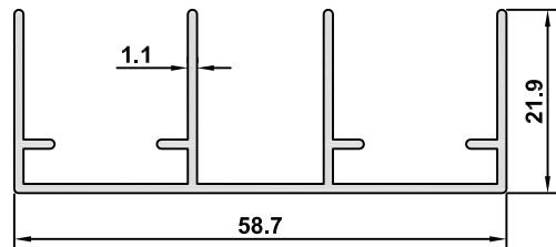
6207 AĞIRLIK / WEIGHT 0,465 kg/m
