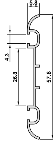
4884 AĞIRLIK / WEIGHT 0,241 kg/m
