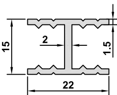
5783 AĞIRLIK / WEIGHT 0,260 kg/m
