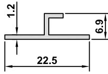
5238 AĞIRLIK / WEIGHT 0,106 kg/m
