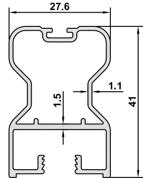
5989 AĞIRLIK / WEIGHT 0,550 kg/m
