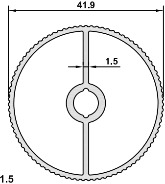
7130 AĞIRLIK / WEIGHT 0,716 kg/m
