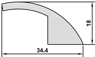
5148 AĞIRLIK / WEIGHT 0,553 kg/m
