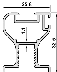
6203 AĞIRLIK / WEIGHT 0,440 kg/m
