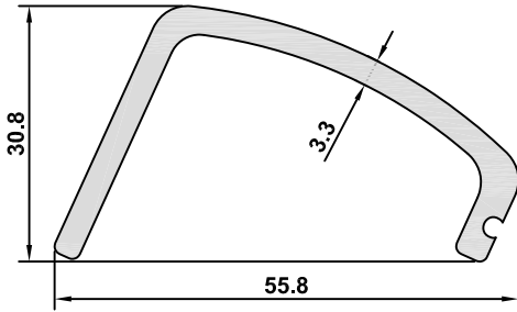
5249 AĞIRLIK / WEIGHT 3,141 kg/m
