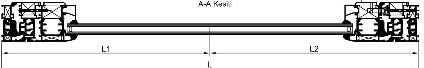
Section A-A A-A Kesiti
