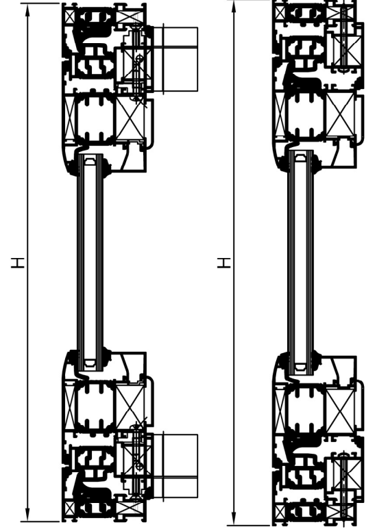
Section B-B B-B Kesiti
