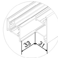
Section A-A A-A Kesiti
