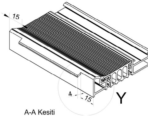
A-A Kesiti Section A-A
