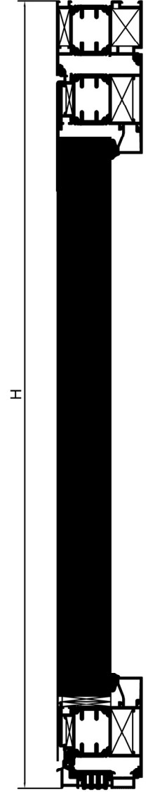
B-B Kesiti Section B-B
