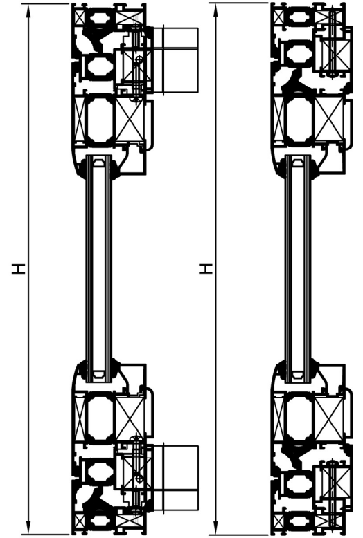
Section B-B B-B Kesiti
