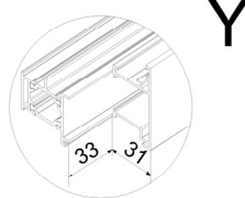
Section A-A A-A Kesiti
